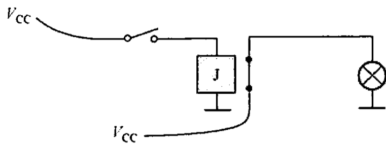
图 7.3 继电器电路的另一种简化形式
