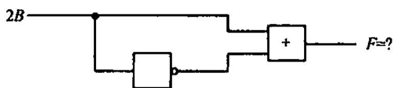
图 5.22 莎士比亚电路
