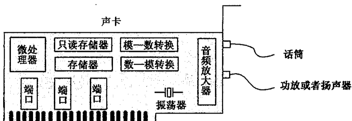
图 14.6 声卡的基本组成
