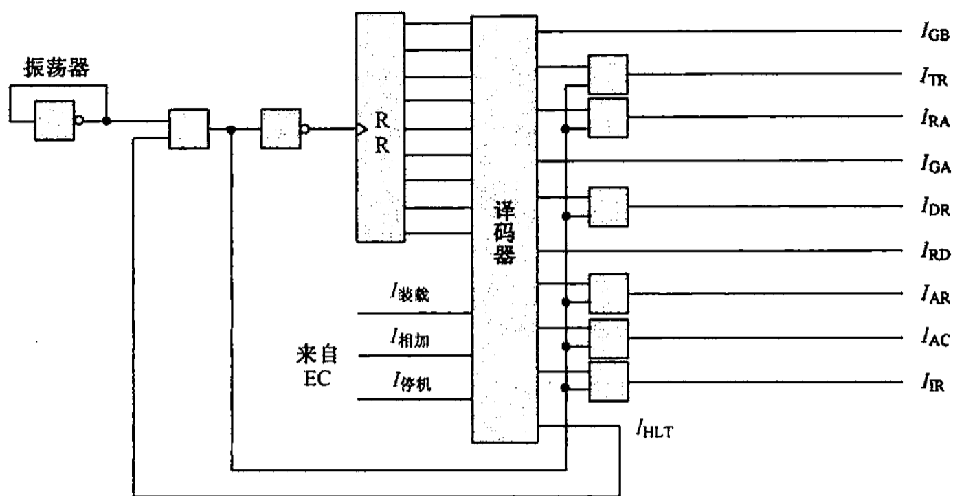
图 11.23 重新设计的控制器
