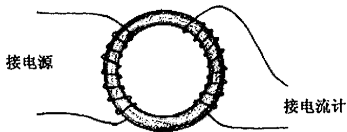
图 4.6 法拉第用来将磁变成电的装置
