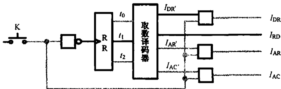
图 11.16 取数控制器的原理 (3)
