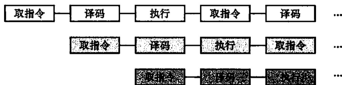
图 13.8 超标量体系结构
