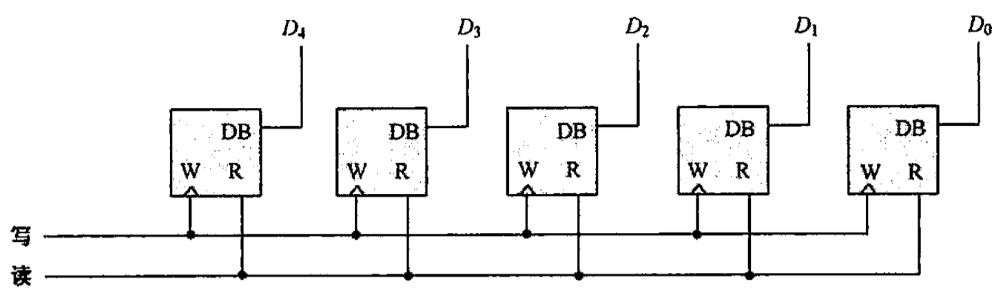
图 11.5 可以读/写单个 5 位二进制数的存储器
