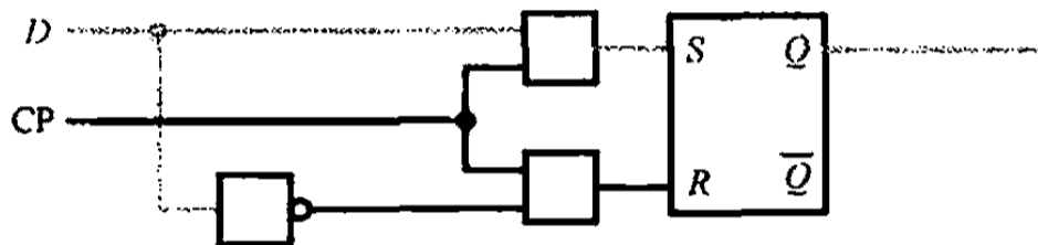
图 8.7 当控制端为 1 时，如果 D 端为 0，触发器的 Q 端为 0
