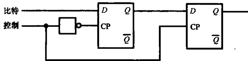
图 8.12 上升沿触发器的原理
