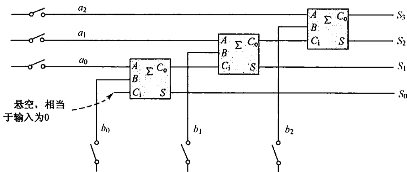
图 3.8 由 3 个全加器组成的 3 比特加法机（结果是 4 比特）
