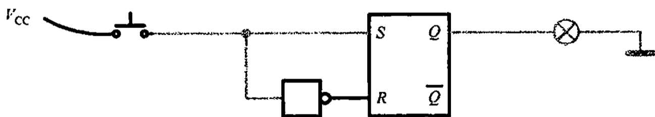
图 8.3 使用触发器保存比特“0”的过程
