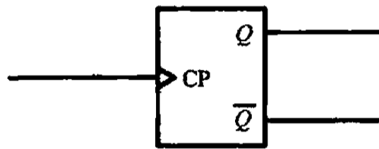
图 9.6 乒乓触发器的符号
