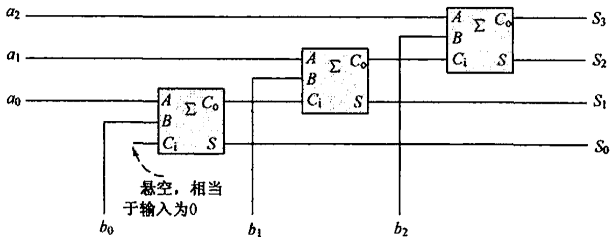
图 6.4 用全加器组成一个三比特加法电路
