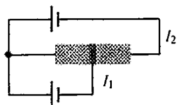
图 9.2 晶体三极管工作原理示意图
