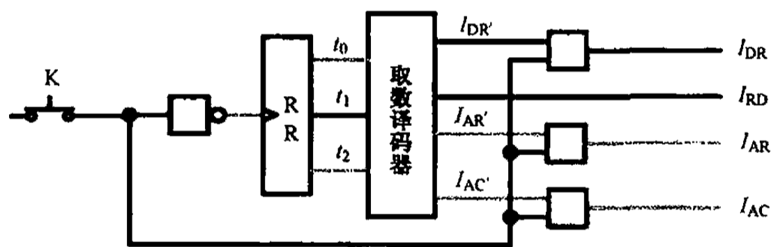
图 11.17 取数控制器的原理 (4)
