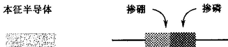
图 9.1 本征半导体的掺杂方法
