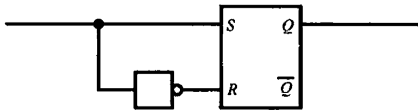
图 8.2 使用非门使 R 与 S 总是相反，解决用触发器保存 1 个比特的问题
