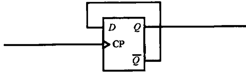
图 9.5 乒乓触发器示意图
