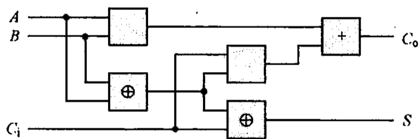
图 6.3 用异或门组成的全加器
