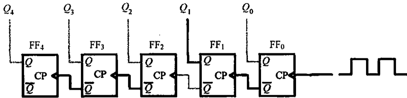
图 9.9 当第二个脉冲到来后，计数器的值为 00010
