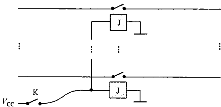
图 10.7 用一只开关来控制多条线路的通断
