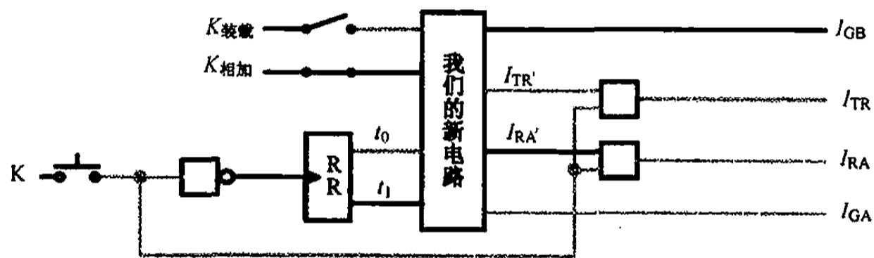
图 10.17 相加过程 (3)
