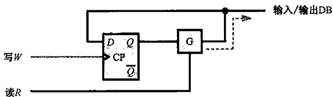
图 11.3 读出一个比特的原理
