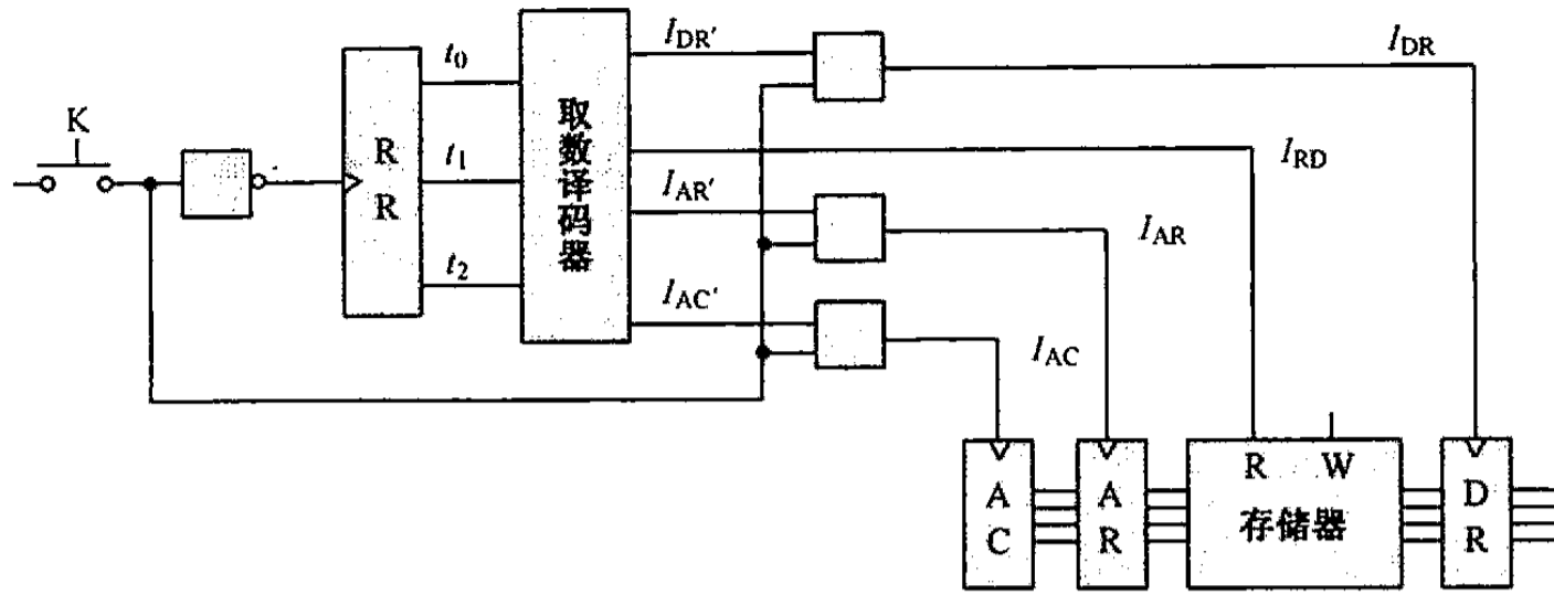
图 11.13 用一只开关依次将数取出
