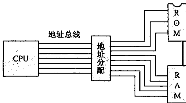
图 15.2 中央处理器的地址空间分配
