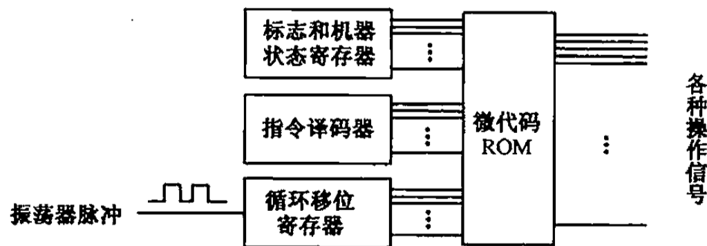
图 13.3 现代计算机的控制器结构
