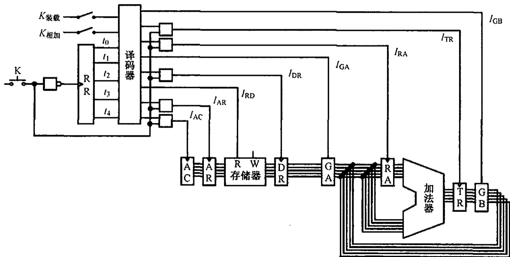
图 11.20 部分实现了自动化的连续加法电路
