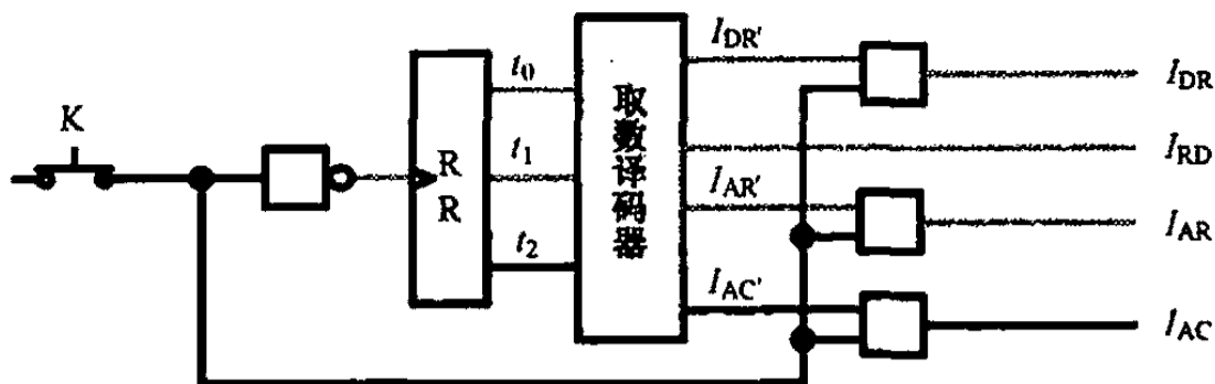
图 11.19 取数控制器的原理 (6)
