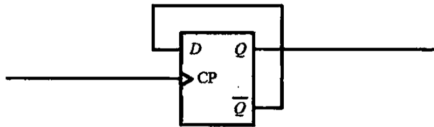
图 8.16 首尾相连的上升沿 D 触发器
