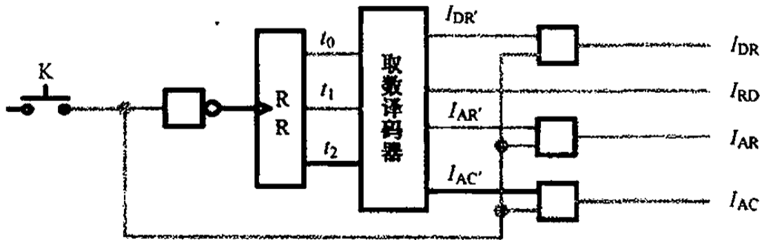
图 11.18 取数控制器的原理 (5)
