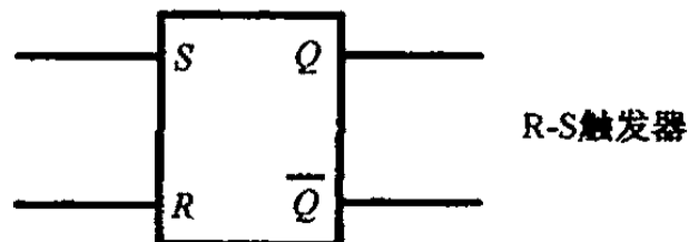
图 7.19 R-S 触发器的符号
