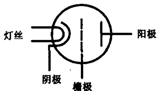
图 7.12 电子三极管的符号
