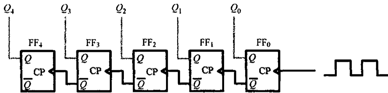
图 9.7 5 个乒乓触发器构成的计数器
