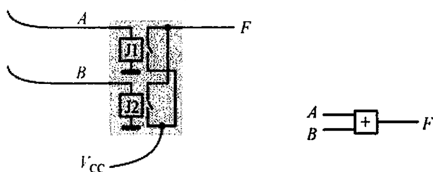
图 5.16 或门及其符号
