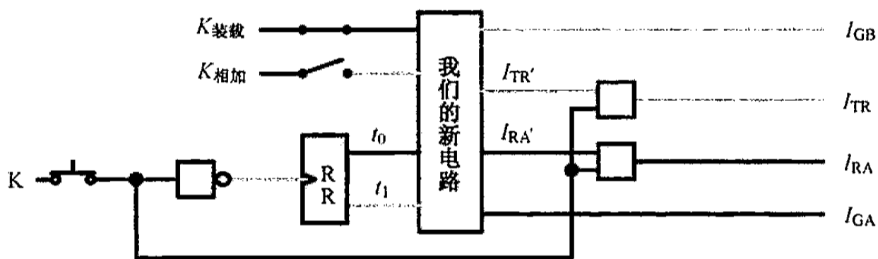
图 10.12 装载数据的过程 (2)
