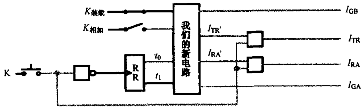
图 10.13 装载数据的过程 (3)
