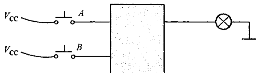
图 7.1 连着两个按键开关的逻辑电路
