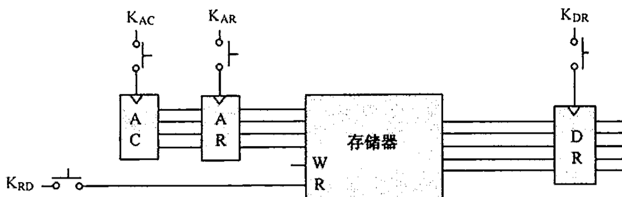
图 11.12 顺序地从存储器里取数的电路方案
