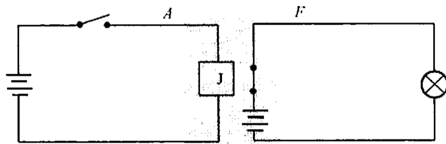
图 5.7 一个应用非门的例子
