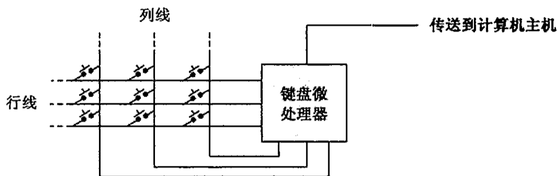
图 14.7 键盘电路
