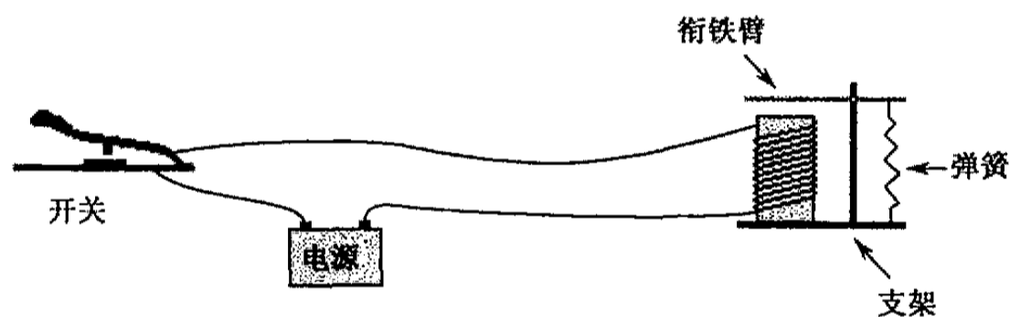
图 4.2 莫尔斯电报示意图
