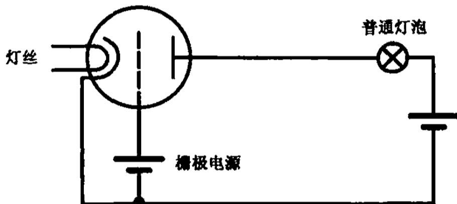
图 7.13 电子三极管的原理示意
