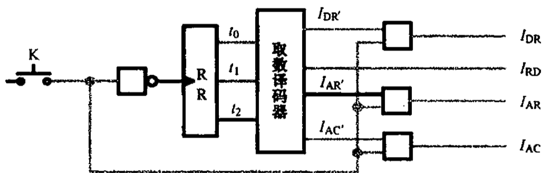
图 11.14 取数控制器的原理 (1)
