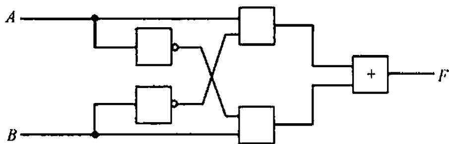
图 5.18 \bar{A}B + A\bar{B} 的逻辑电路组成
