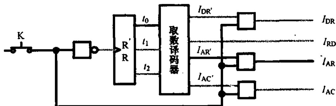
图 11.15 取数控制器的原理 (2)
