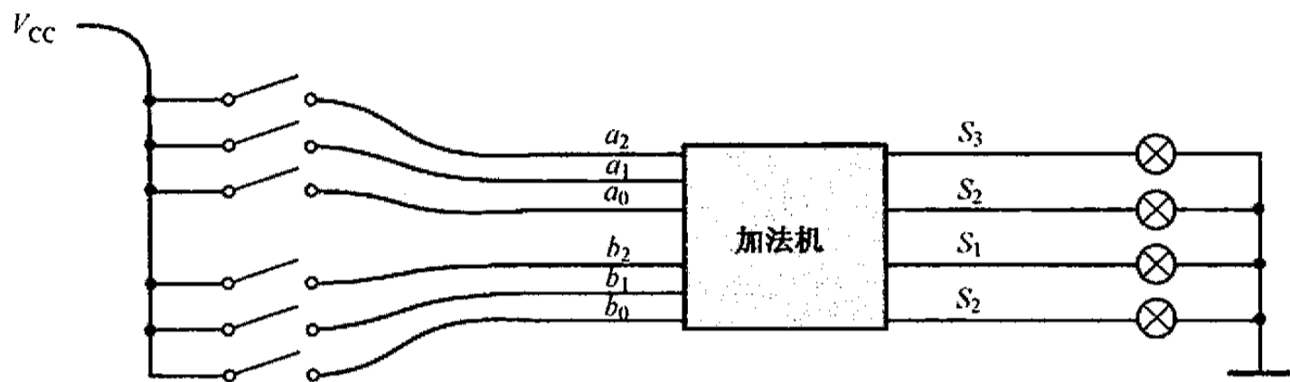
图 6.6 加法机电路的完整连接图
