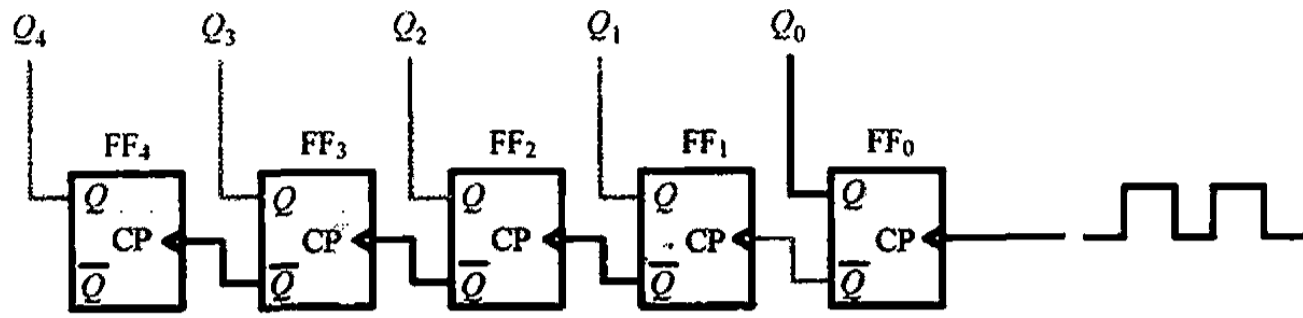
图 9.8 当第一个脉冲到来后，计数器的值为 00001
