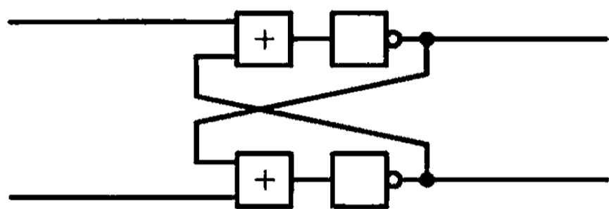
图 7.14 两个或非门首尾相连形成两个反馈
