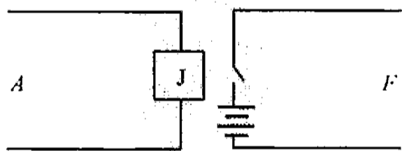
图 5.5 一个自带电源的继电器
