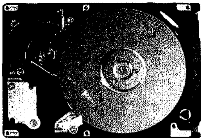
图 15.4 硬盘的内部构造
