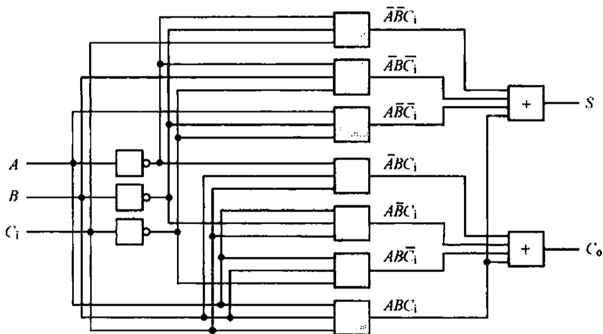
图 6.2 全加器的逻辑电路实现
