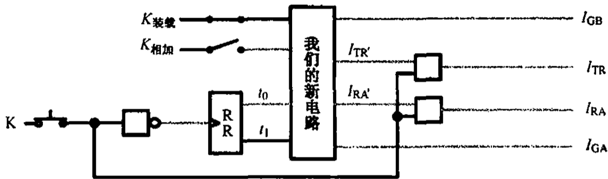
图 10.14 装载数据的过程 (4)
