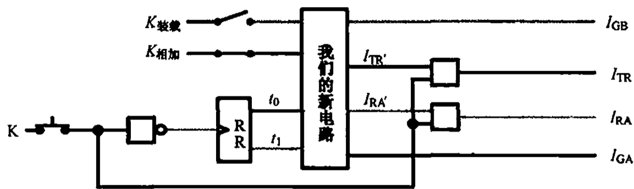
图 10.16 相加过程 (2)
