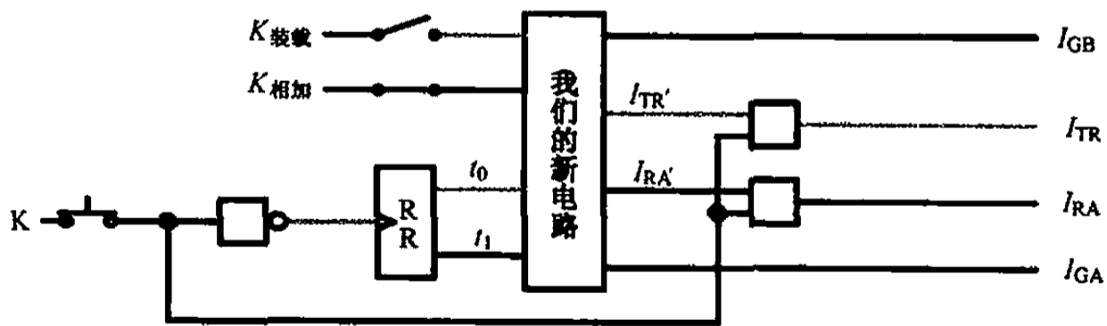
图 10.18 相加过程 (4)
