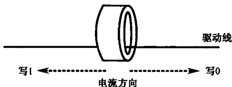
图 11.9 电流方向决定了磁芯的磁化方向
