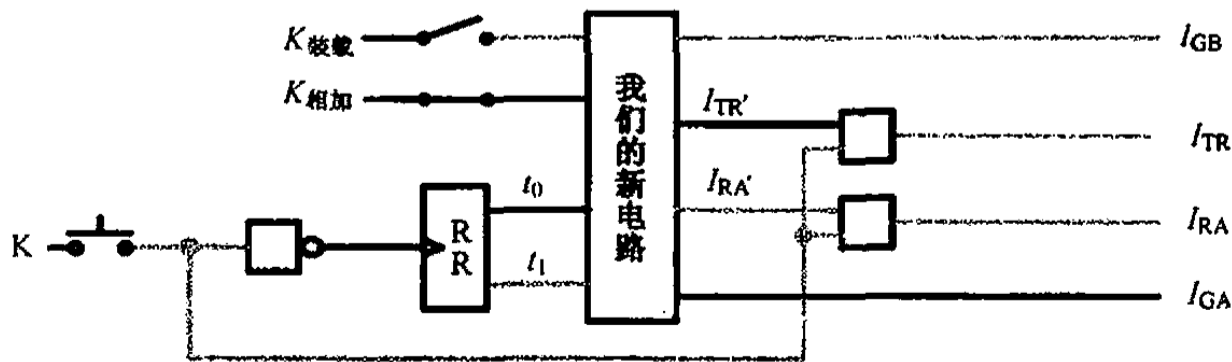
图 10.15 相加过程 (1)
