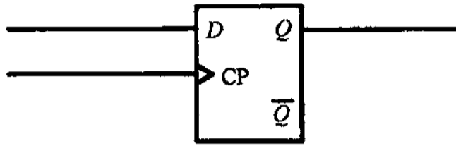
图 8.13 上升沿 D 触发器的符号
