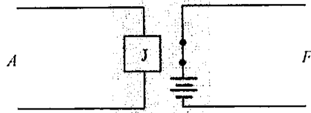
图 5.6 一个自带电源的常闭触点继电器属于非门
