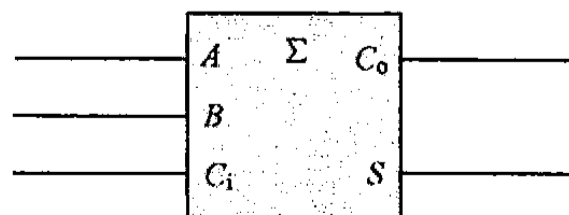
图 3.7 全加器示意图
