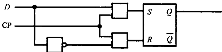
图 8.5 经过改进的触发器，增加了 1 个控制端
