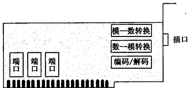
图 14.4 计算机接口卡的外观和基本组成
