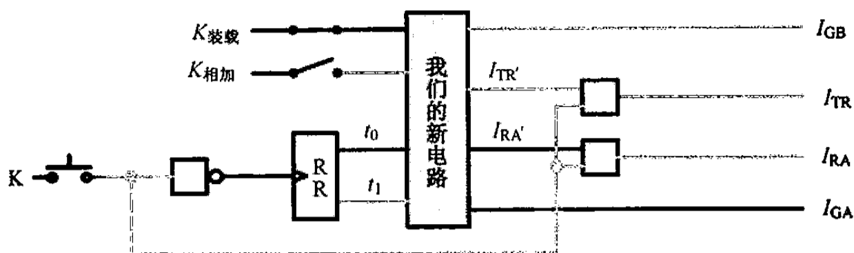
图 10.11 装载数据的过程 (1)
